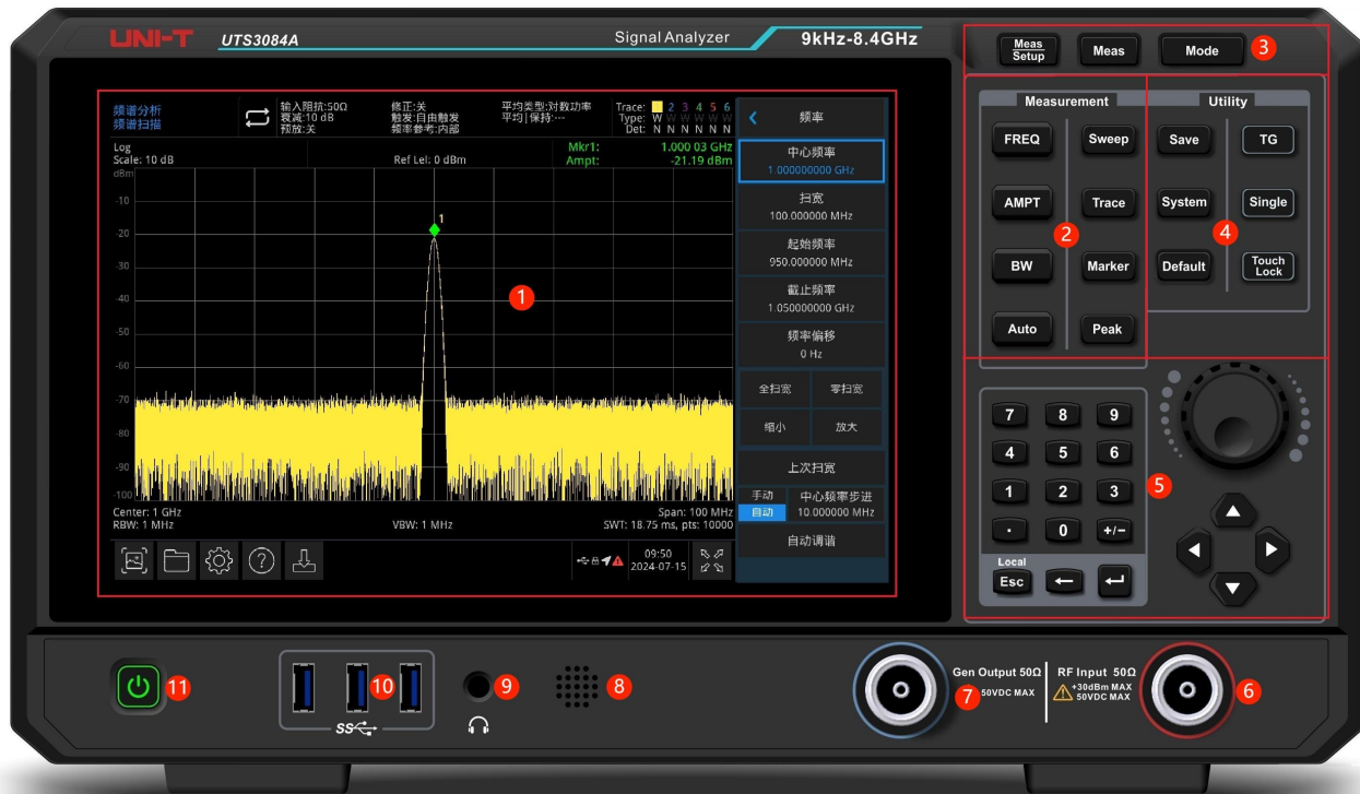
图 1-1: 前面板
