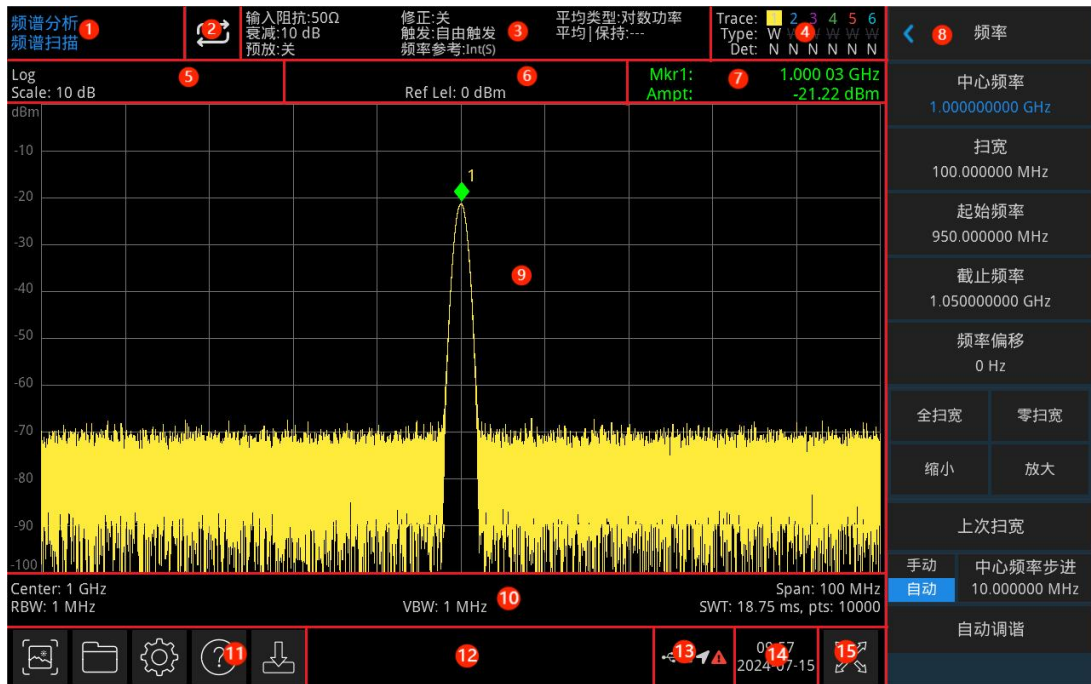
图 1-2: 用户界面
