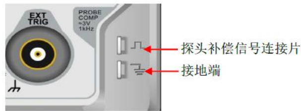
图 1 探头补偿信号连接片和接地端
