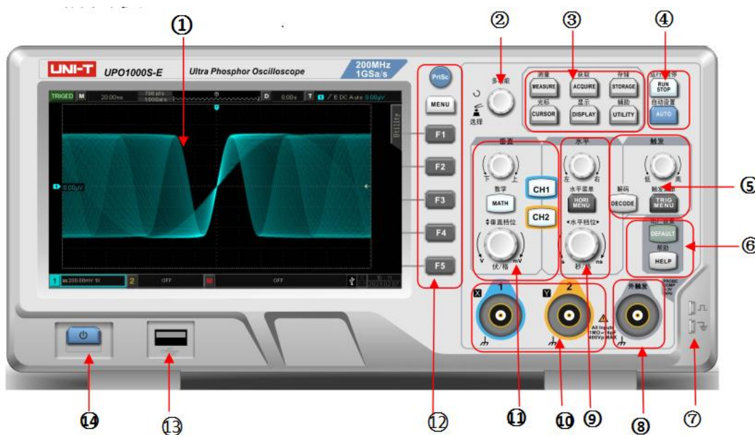
图 4-3 示波器前面板
