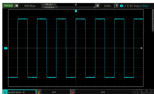
采用 32 次平均的波
