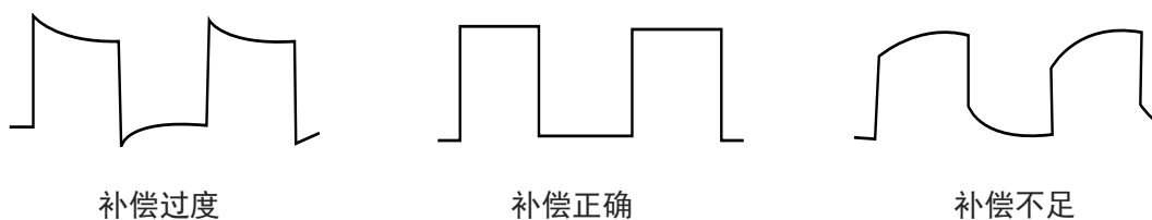
图 4-2 探头补偿校正
