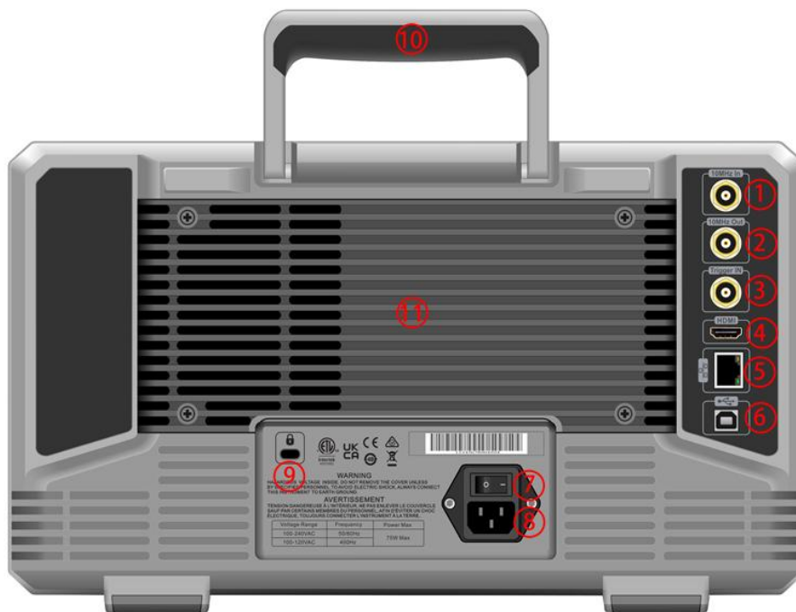
图 1-3: 后面板
