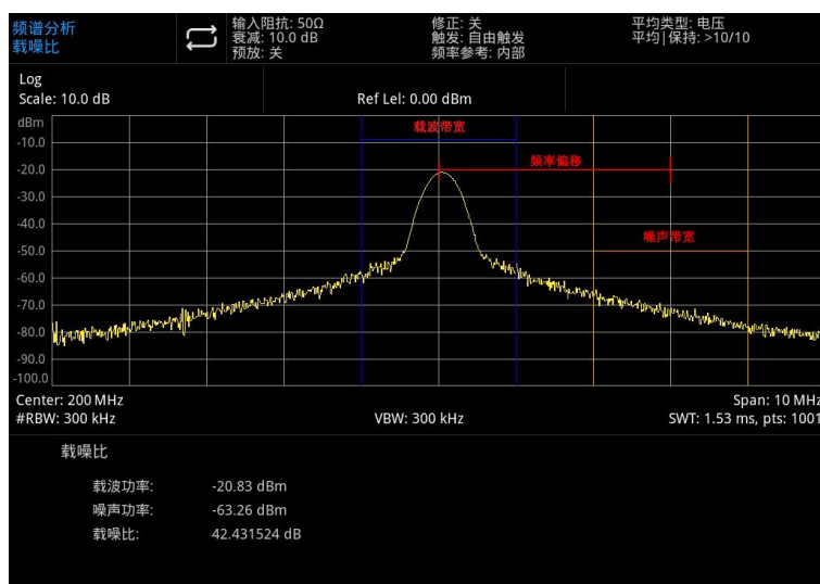
图 5-7：载噪比测量
