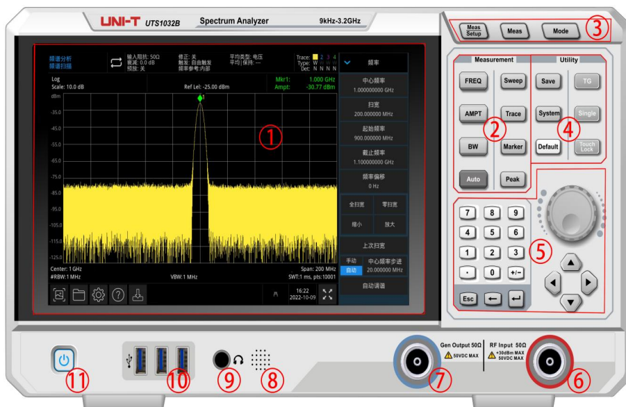
图 1-1: 前面板
