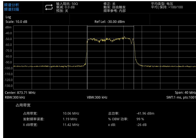
图 5-3:占用带宽
