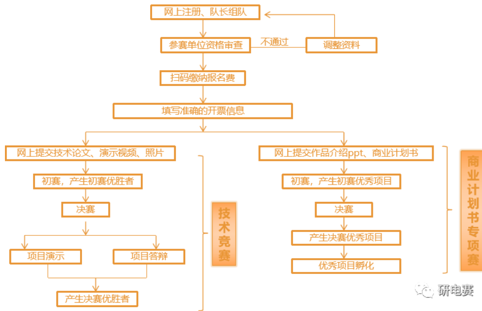
参赛流程图
